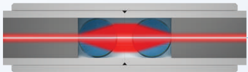
Expanded Beam Verbindung
