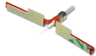
1.25 mm / 2.5mm Ferrulen-Baugruppe (Krokodil Fusion-Alberino)
