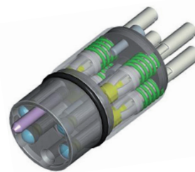
Module interne X-BEAM 4 canaux
